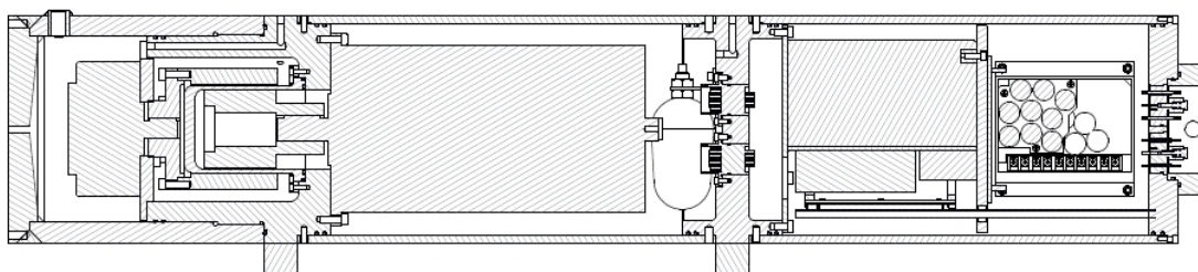
Tverrsnitt
